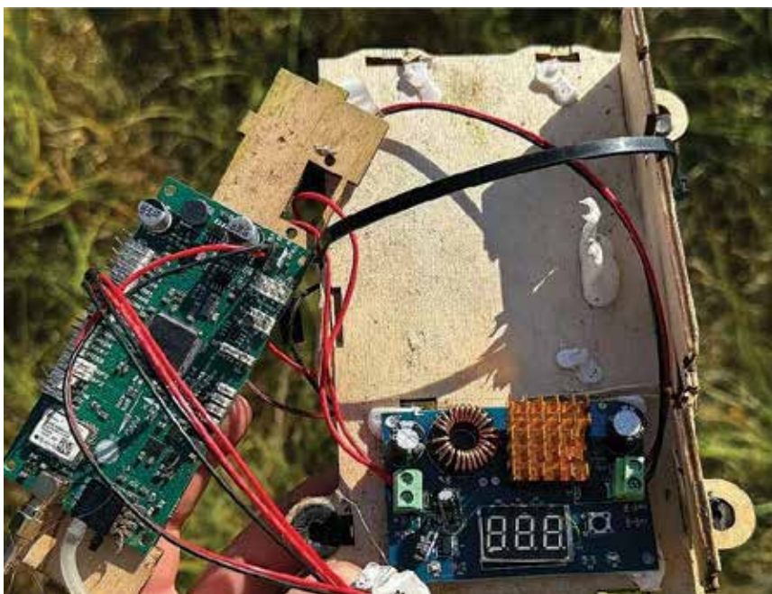
Elektroninės įrangos dalis, rasta numušto drono Gerbera nuolaužose. Gerai matyti fanerinio vidinio įdėklo likučiai.
